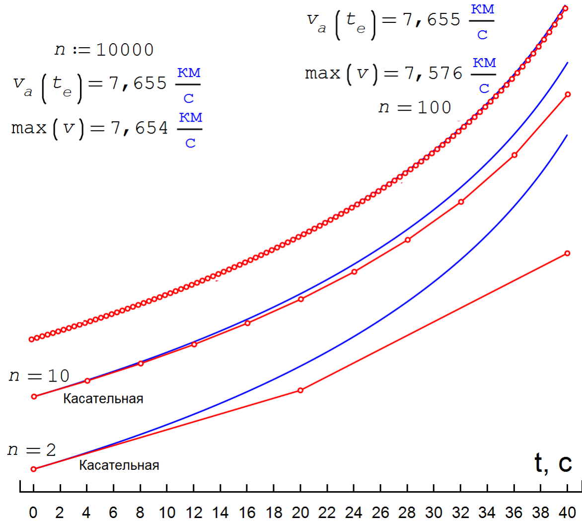
Рис. 10.4. Ломанные Эйлера
